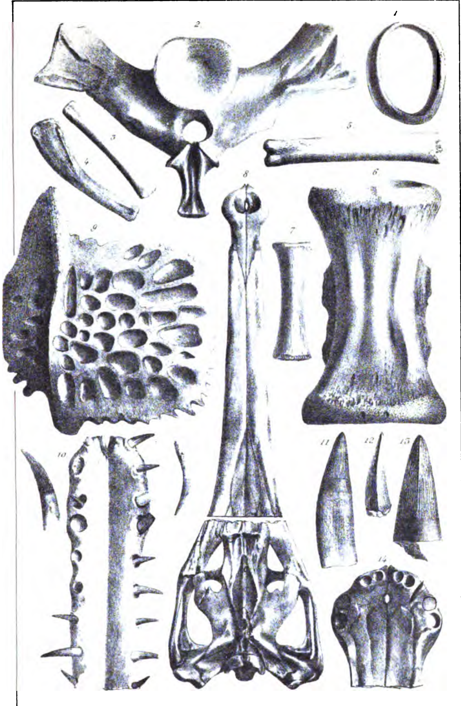
Auonstadt, Jura.
